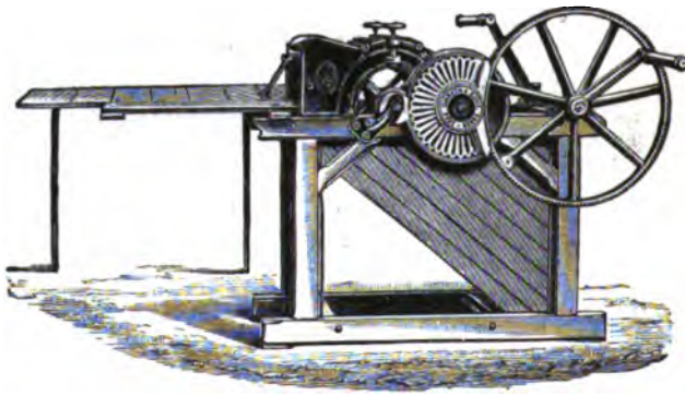
7. Ruční mlatička kolková.
